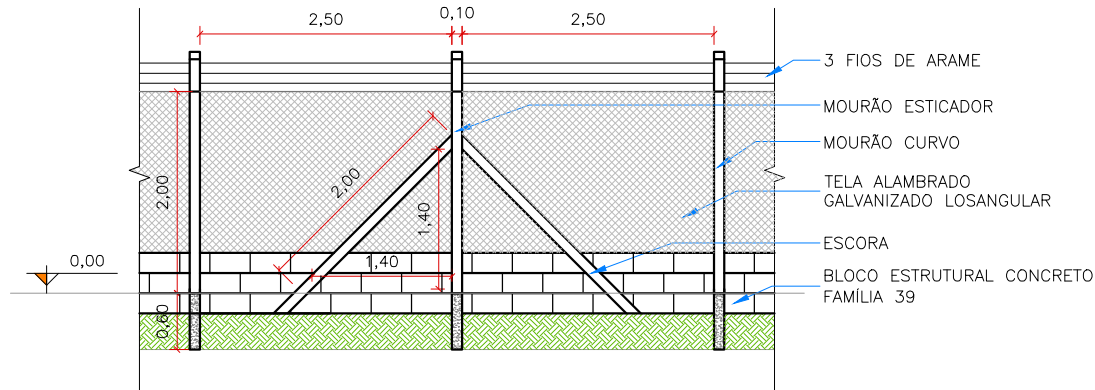
DETALHE: MOURÃO ESTICADOR COM ESCORAS
