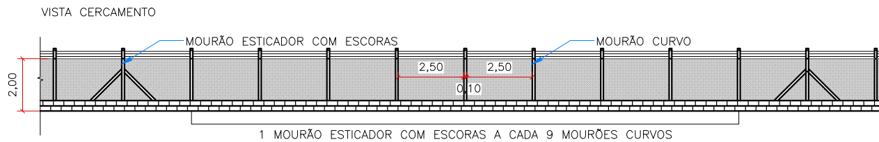
A DETALHE MOURÃO CURVO E MOURÃO ESTICADOR – Esc.:1/75
