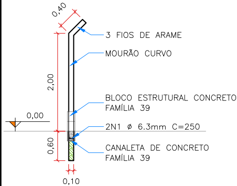
A DETALHE MOURÃO CURVO E MOURÃO ESTICADOR – Esc.:1/75
