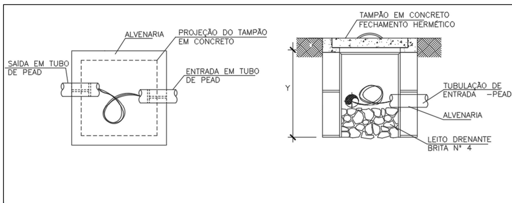
Figura 01: Detalhamento de projeto
