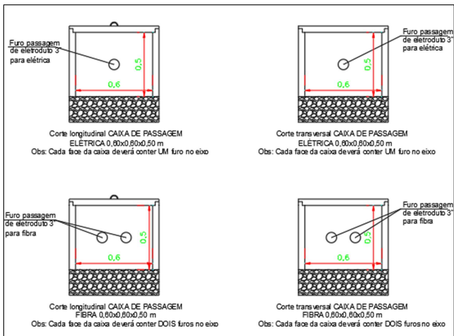
Figura 03: Representação dos furos circulares nas caixas de elétrica e fibra (lógica) dimensão 0,60x0,60x0,50m
