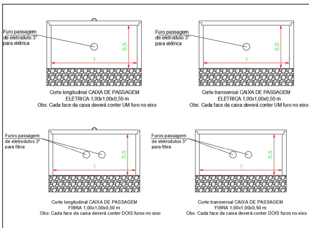
Figura 02: Representação dos furos circulares nas caixas de elétrica e fibra (lógica) dimensão 1,00x1,00x0,50m
