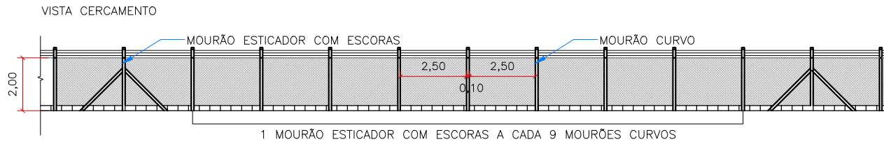
A DETALHE MOURÃO CURVO E MOURÃO ESTICADOR – Esc.:1/75
