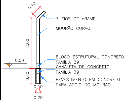
A DETALHE MOURÃO CURVO E MOURÃO ESTICADOR – Esc.:1/75
